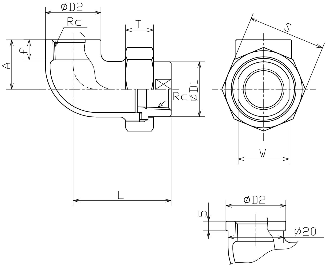
ユニオンエルボ（8Aのみ）
